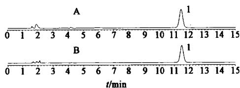
A. 对照品; B. 供试品; 1. 青蒿琥酯 图 1 青蒿琥酯原料药 HPLC
