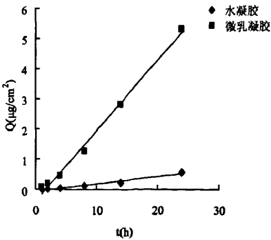
图 4 两种凝胶中吴茱萸碱经皮渗透曲线
